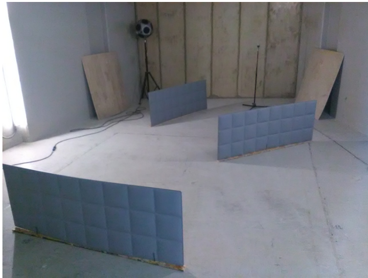
Figura 6_Camera Riverberante con Campioni
